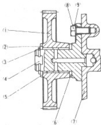
Fig. 36. Idler Gear
