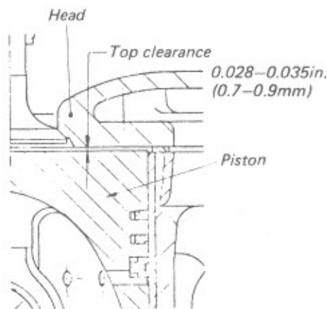
Fig. 21. Top Clearance
